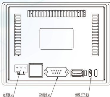
背视图
